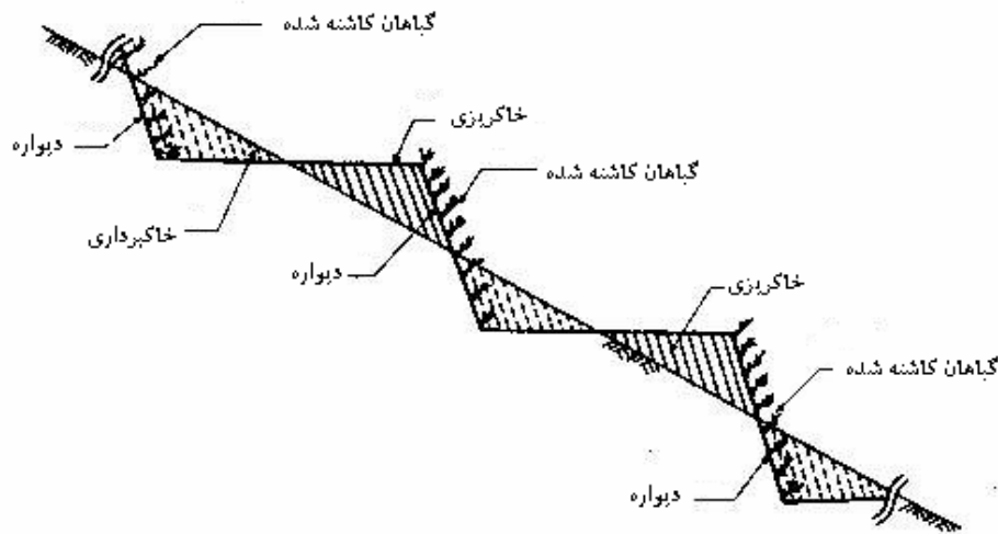
شکل شماره ۱۲ نحوه کاشت گیاه بر روی دیواره تراس سکویی
